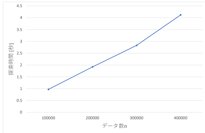
図 1. 線形探索法での探索時間 (文字列 zoozoo を探索)
