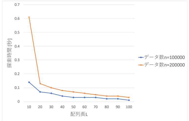
図 2. ハッシュ法での探索時間 (文字列 zoozoo を探索)
